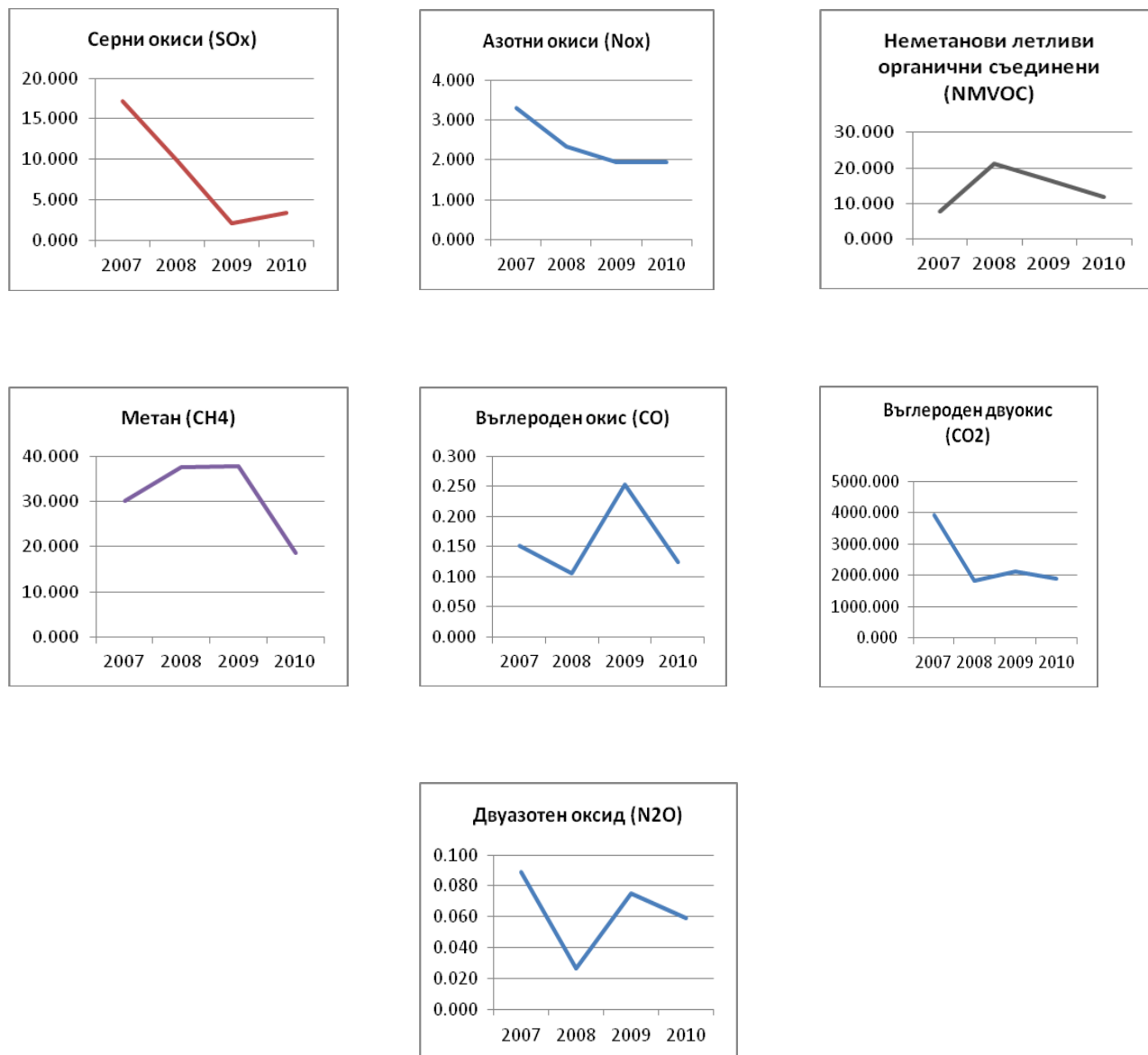
Фигура 34 - Емисии на вредни вещества в атмосферата от горивни и производствени процеси в община Гоце Делчев през периода 2007-2010 г.
